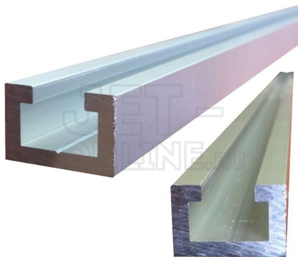
Профиль-шина 19 мм., анод., серебро матовое, 1.0 м.
